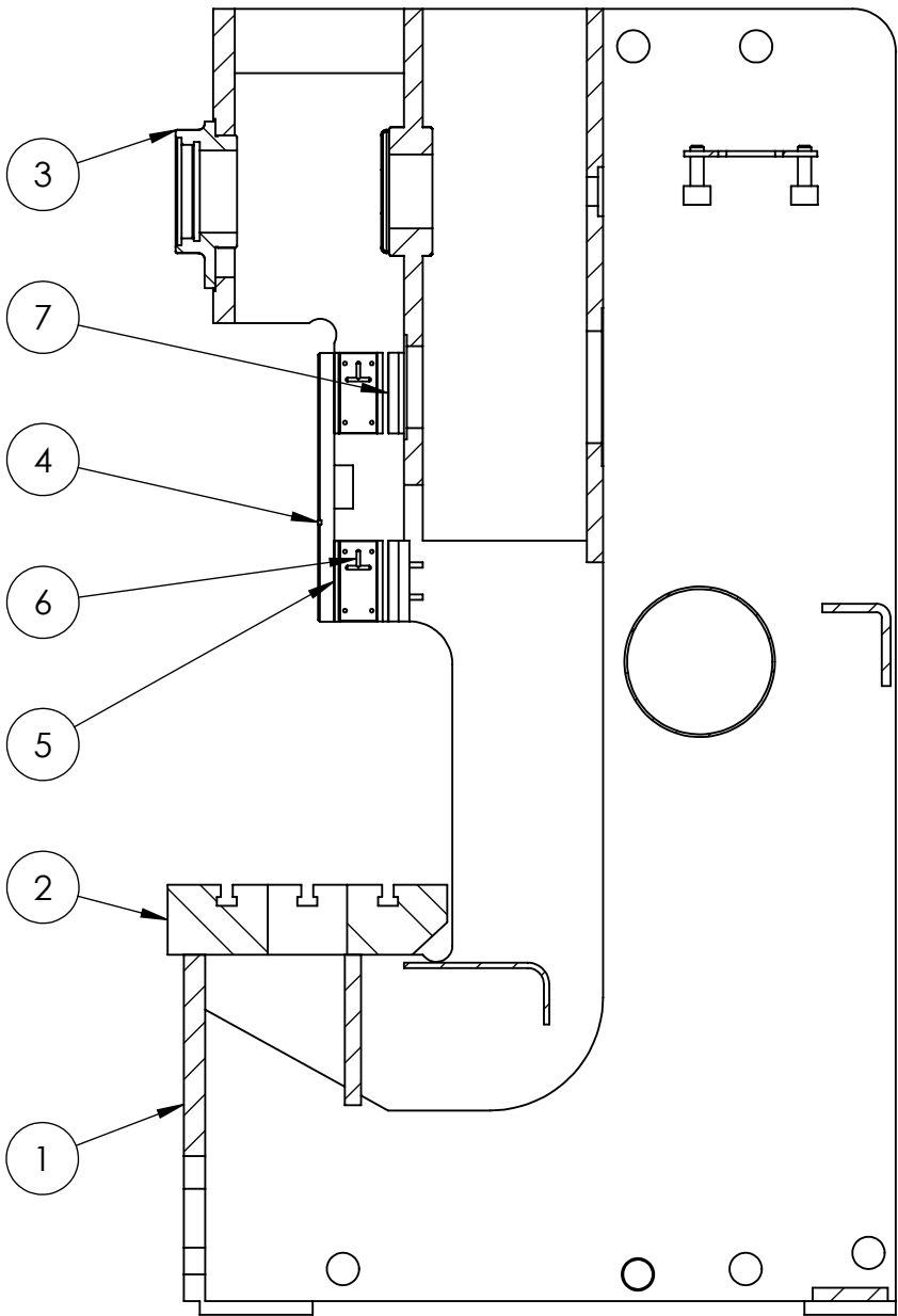
SECTION A-A
